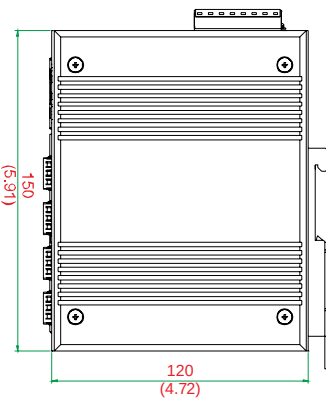
前视图
