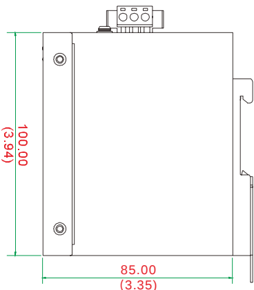
左侧视图
