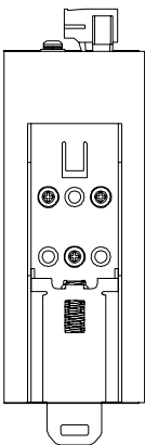
后视图
