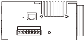
顶视图
