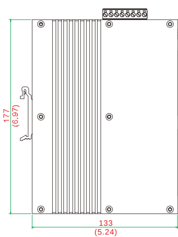
前视图
