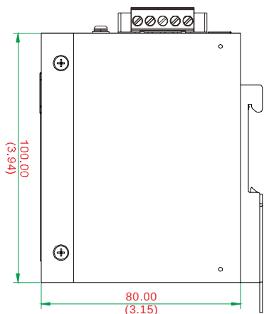
左侧视图
